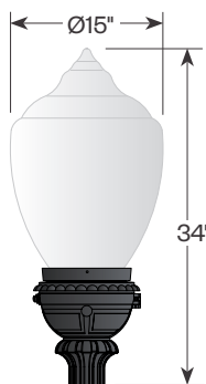
DUF34-AP24
