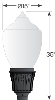
DUF1-AP24
