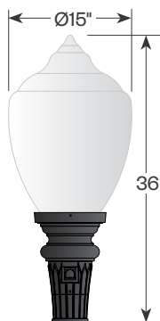
DUF37-AP24
