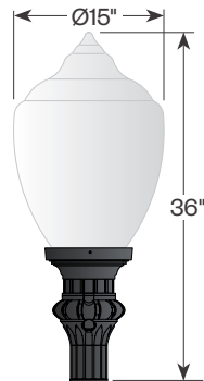
DUF4-AP24
